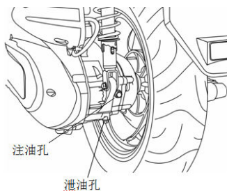
泄油孔
